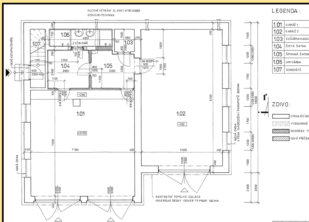
Půdorys 1.NP - nový stav
