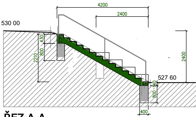
ŘEZ A-A
