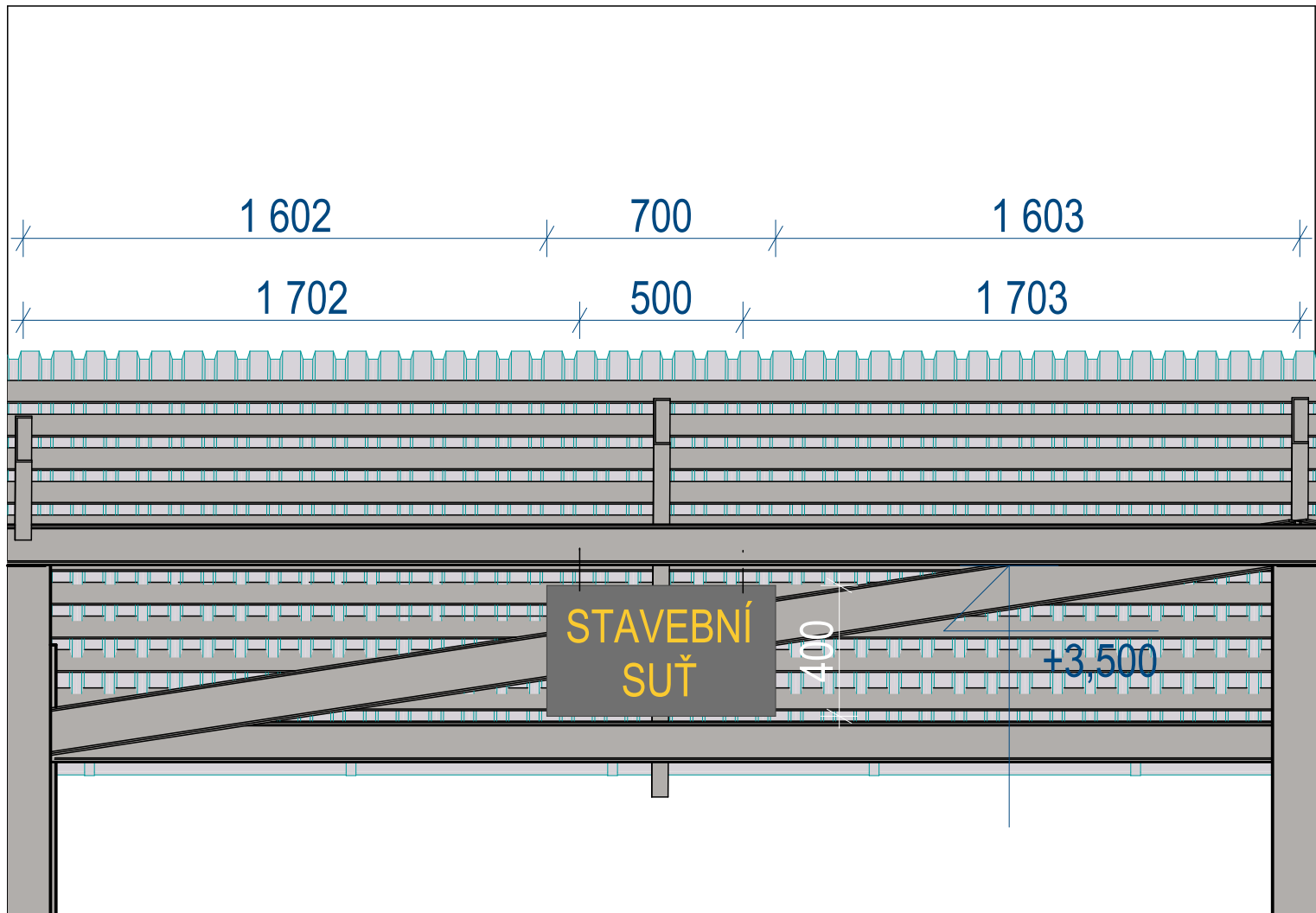
NÁPIS - DETAIL
