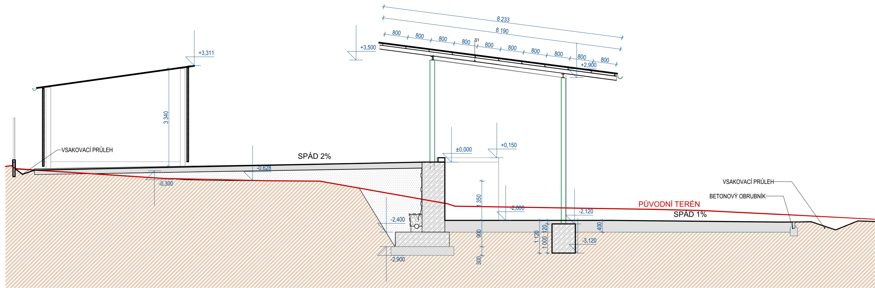
A ŘEZ příčný
