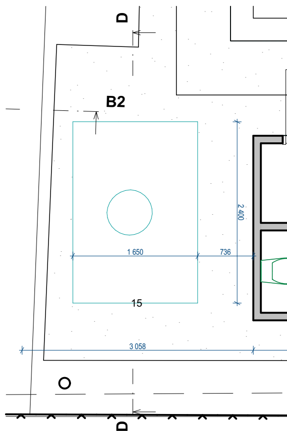
1. PŮDORYS JÍMKY 1:50
