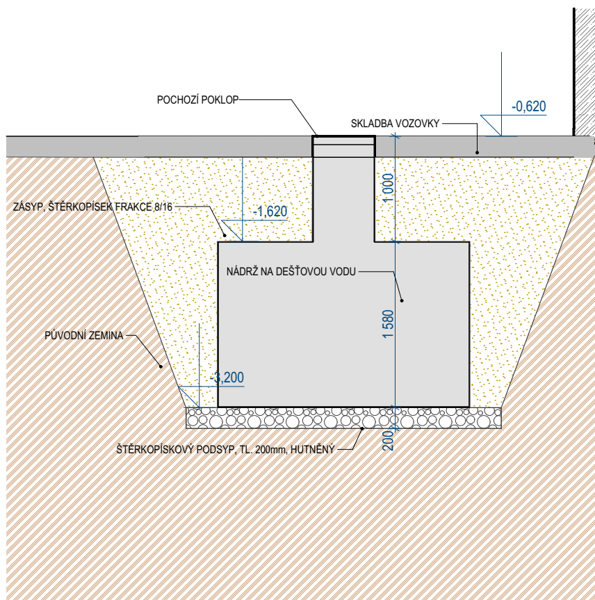
D ŘEZ NÁDRŽÍ 1:50
